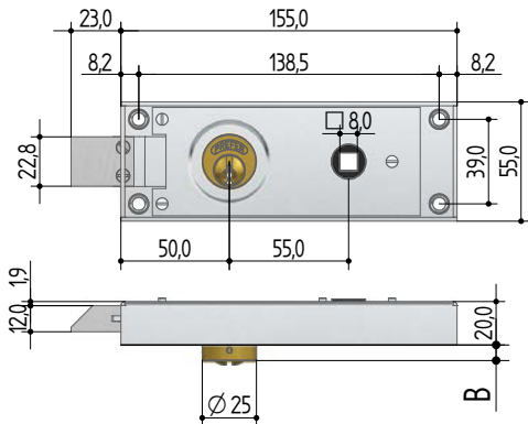
6752 Scrocco rettangolare (2 chiavi dotazione) Square spring latch (2 keys supplied)
